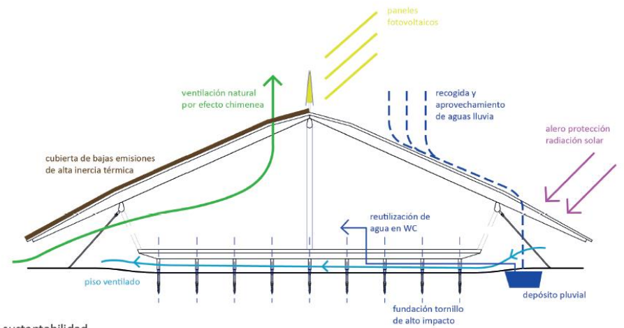
estrategias de sustentabilidad
